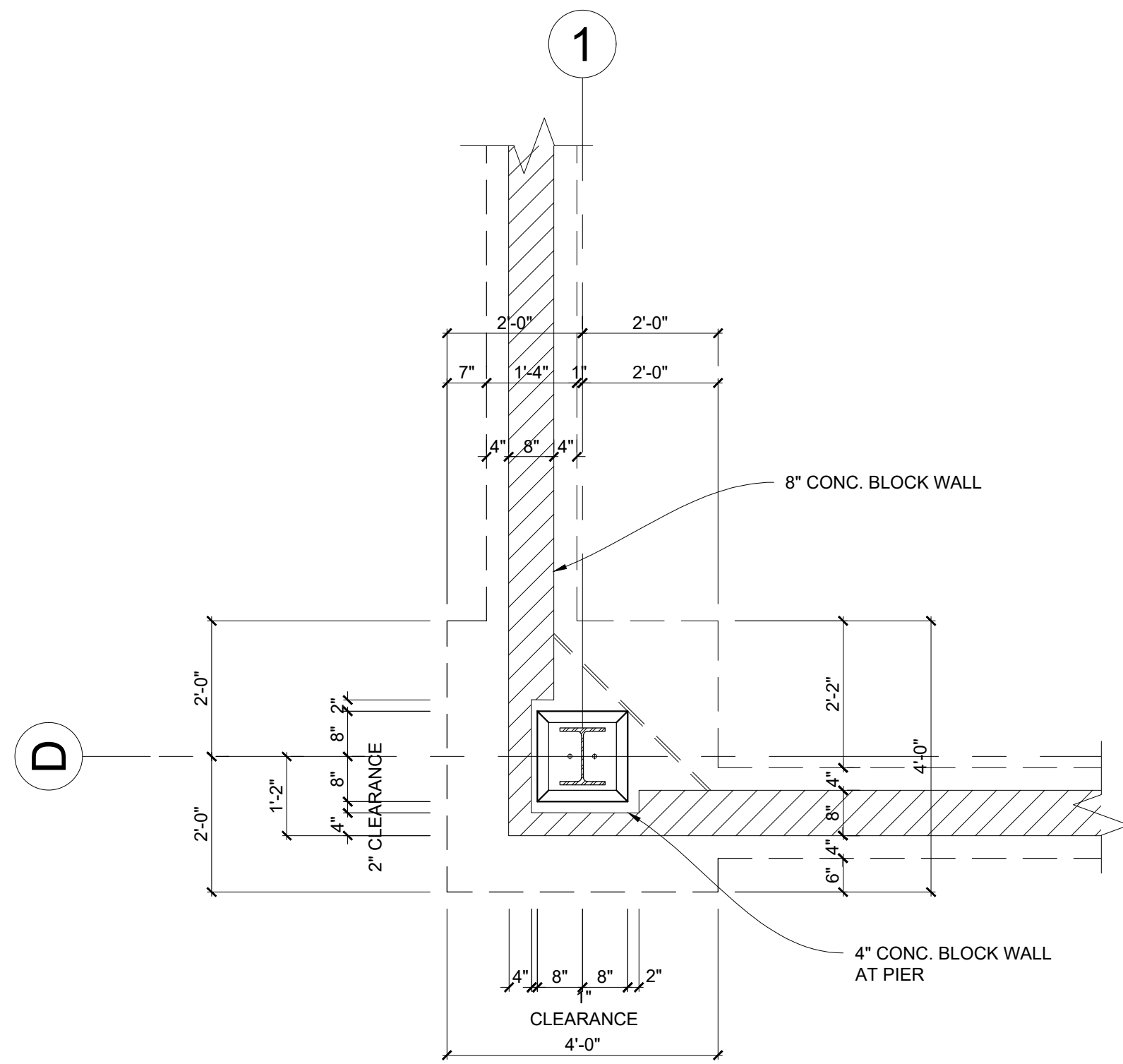
2 FOUNDATION D1 DETAIL SCALE: 1/2" = 1' - 0"
